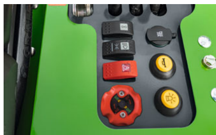
Batteriisolator 1
