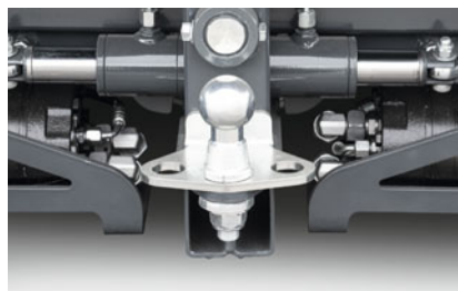
Aanhangerkoppeling, hier met bevestigingspunt 2+3
