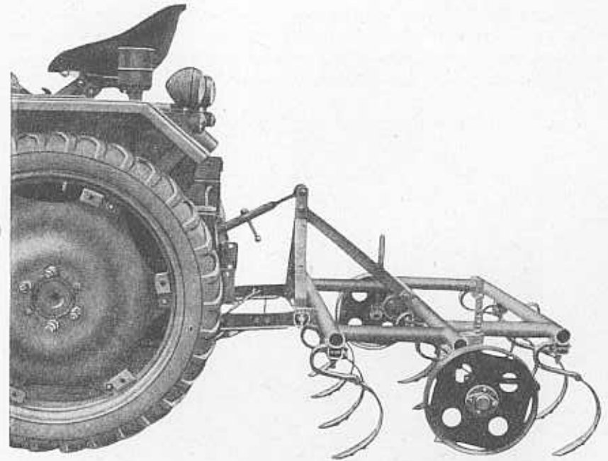
Abb. 1 Anbaugrubber Typ B 233
