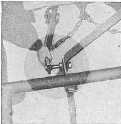
Abb. 6 Befestigung des linken unteren Lenkers
