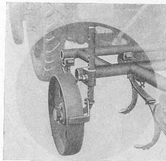
Abb. 8 Stützrad, links
