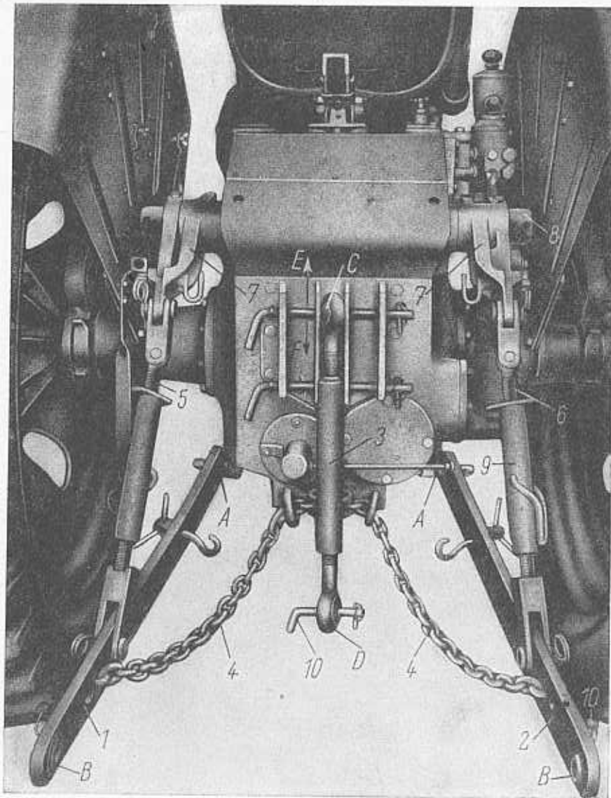
Abb. 5 Dreipunktanbau
