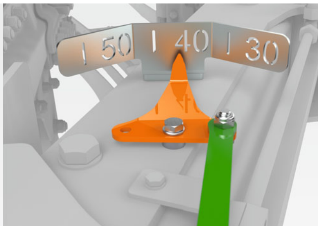
Hydraulische Einstellung der Arbeitsbreite
