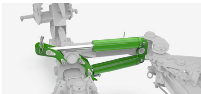
Wendezylinder mit hydraulischer Drossel
