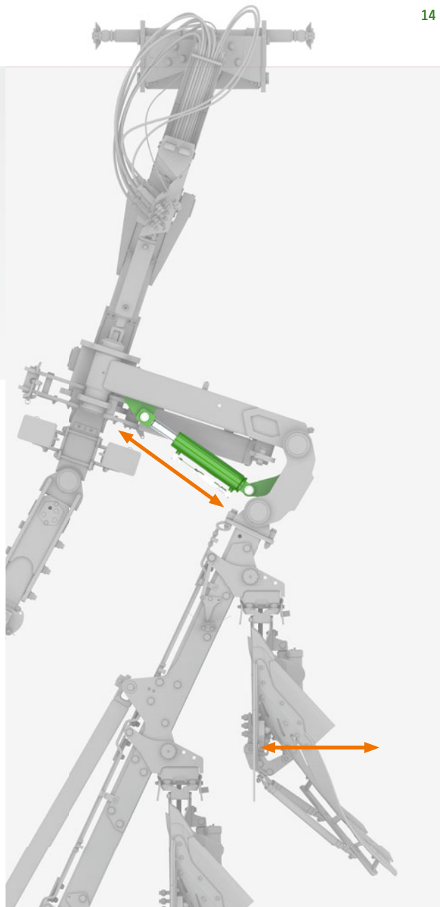
Intelligentes Kinematiksystem zur Anpassung der Vorderfurchenbreite
