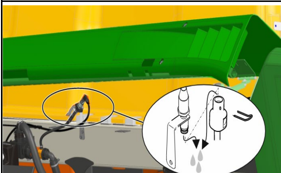
Czujnik ciśnienia mieszadła pod prawa strona za osłoną
