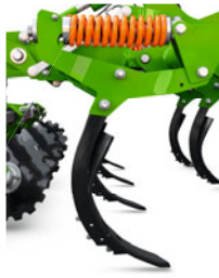
C-Mix-Super-Zinken Mit automatischer Überlastsicherung. Mit 450 kg Auslösekraft – Konzipiert für härteste Bedingungen
