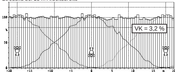
Streubild bei 18 m Arbeitsbreite
