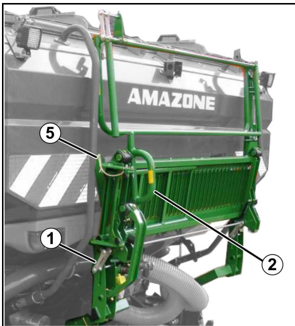
Plnicí lávka v přepravní poloze
