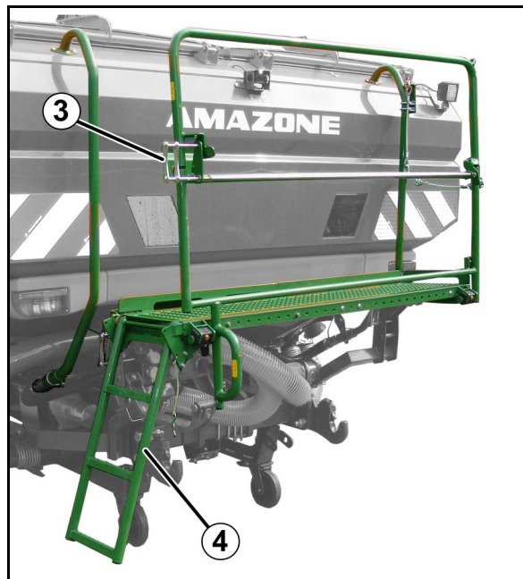
Plnicí lávka v pracovní poloze
