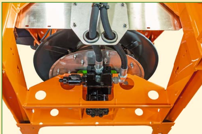
Hydraulischer Streuscheibenantrieb mit streustoffschonendem Rührwerk
