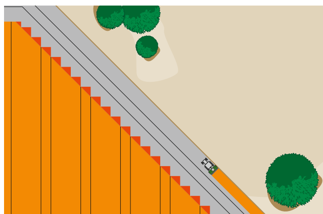
Positionsabhängiges automatisches Ein- und Ausschalten des elektrischen Dosierers mit GPS-Switch
