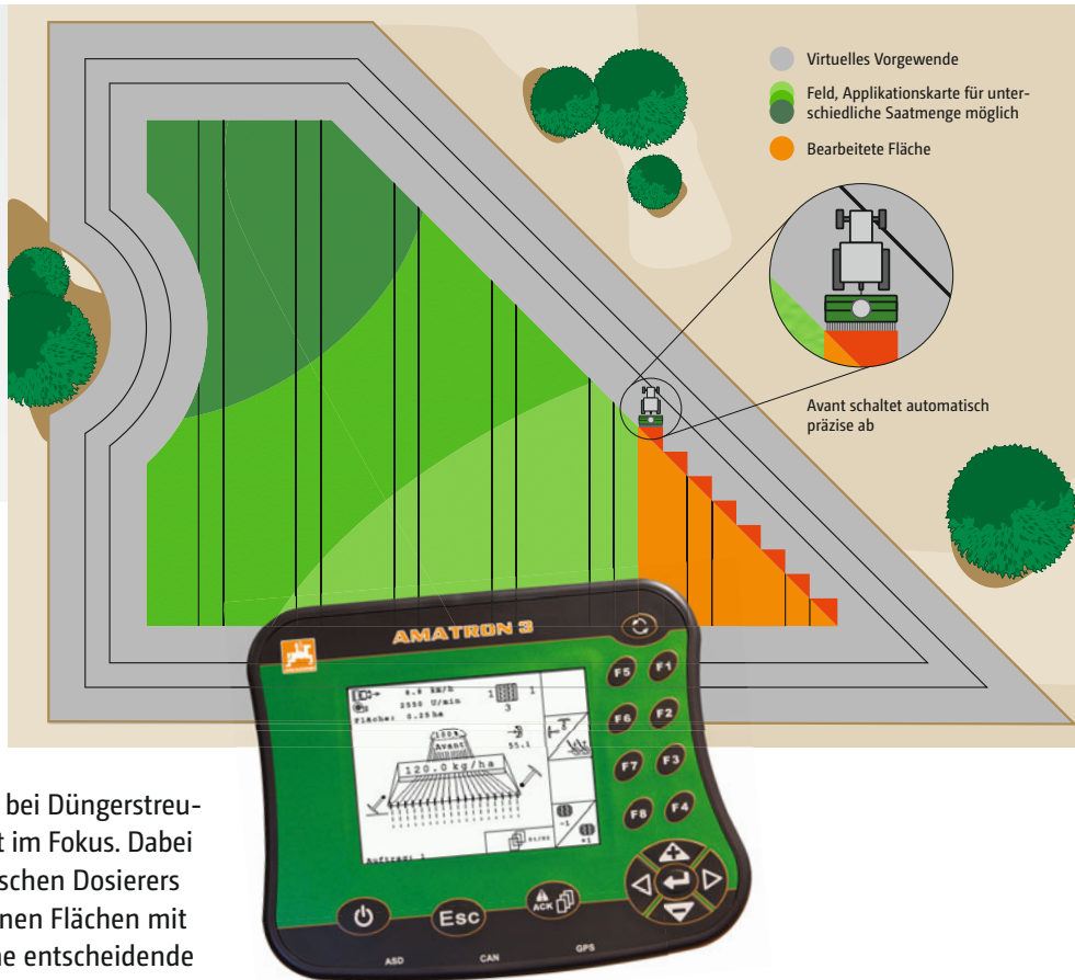
AmaTron 3 für Avant
