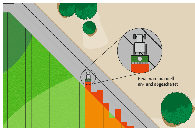
Über- oder Untersäen bei manueller Schaltung ohne GPS-Switch
