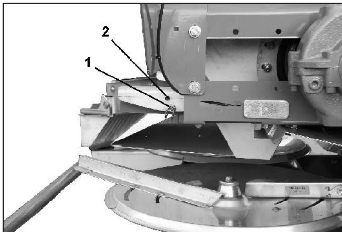
Fig. 7: Omnia-Set-tallrikar „OM“ med fallränna
