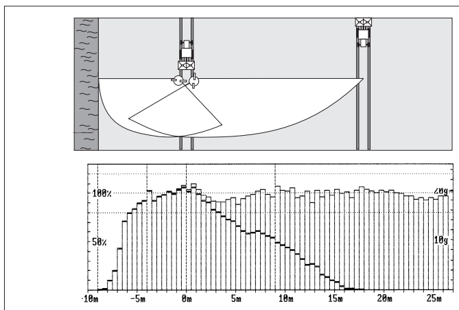
Fig. 20: Vy ovanifrån: miljöoptimerad kantspridning och spridningsbild
