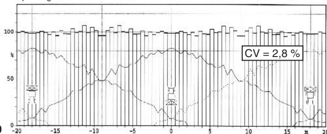
Spridningsbild vid 20m arbetsbredd
