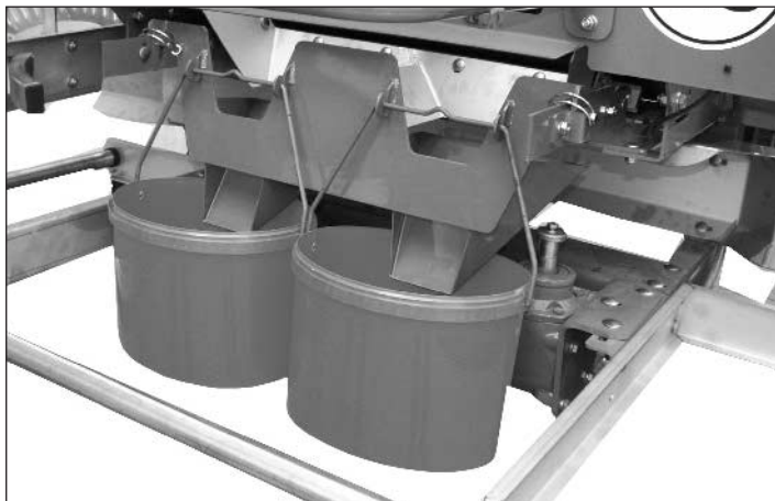
Fig. 3: Bild på mängdprovsningsutrustning
