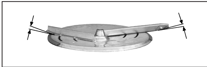
Fig. 9: OM-tallrikar för övergödsling (utkastarvinge uppfäld)
