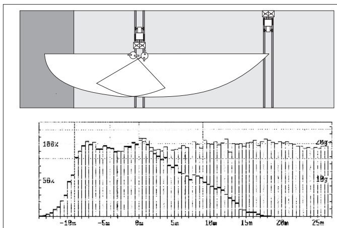
Fig. 21: Vy ovanifrån: skördeoptimerad kantspridning och spridningsbild
