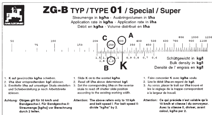
Fig. 1: Beräkningsskivans främre sida (MH11)
