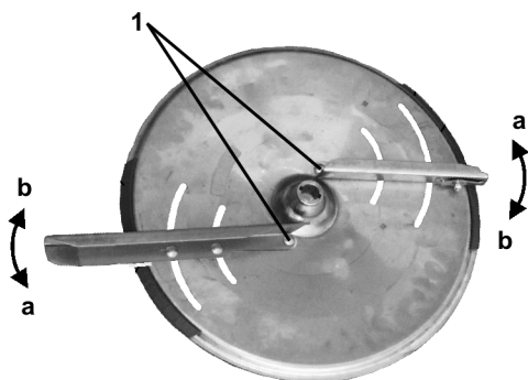
Fig. 13: OM-tallrikar, vy ovanifrån
