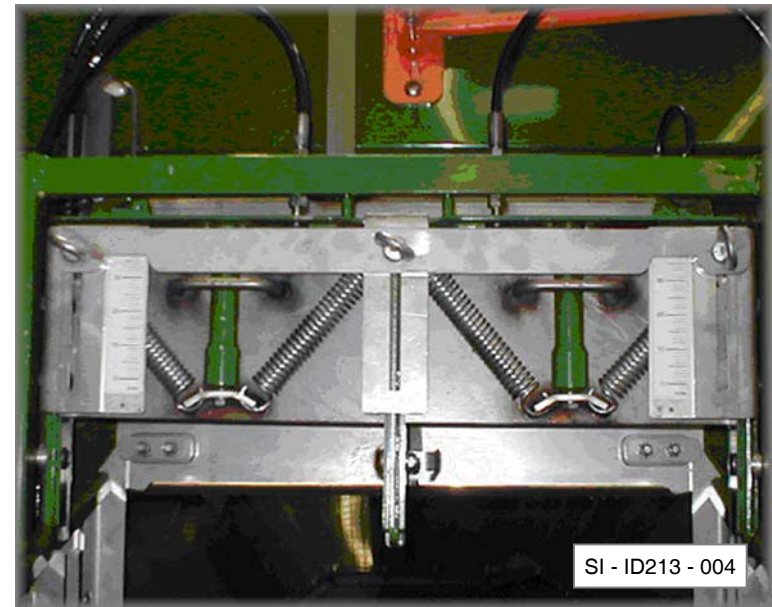
Doppelschieber ZG-B hydraulisch in Parkposition
