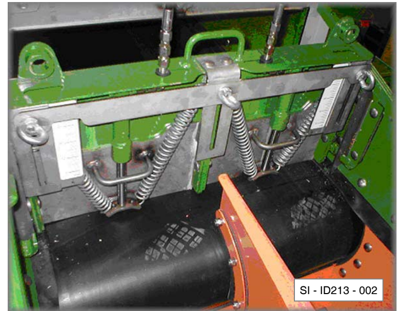
Doppelschieber ZU
