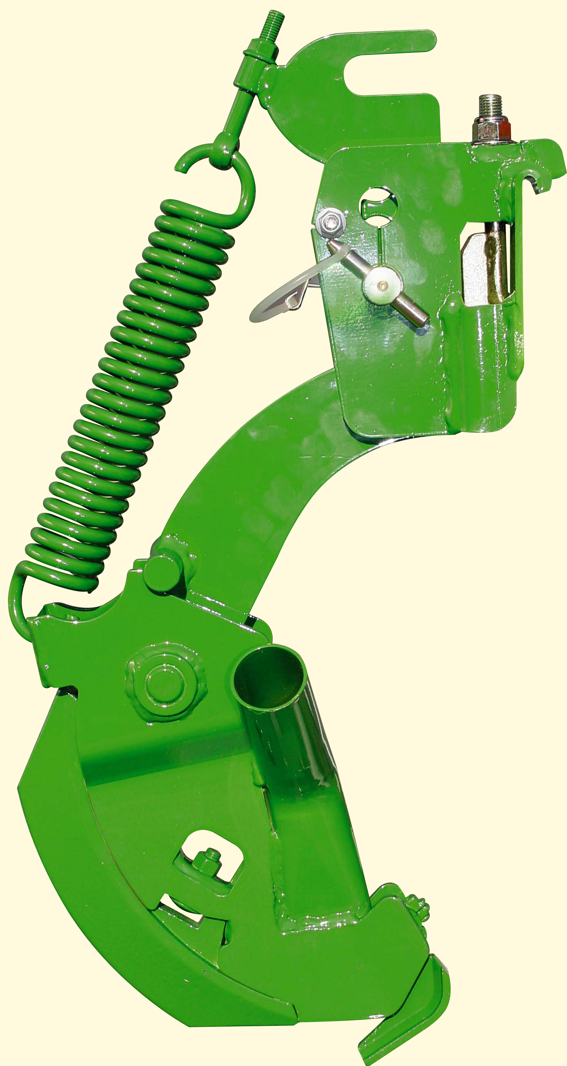
Schleppdüngerschare
