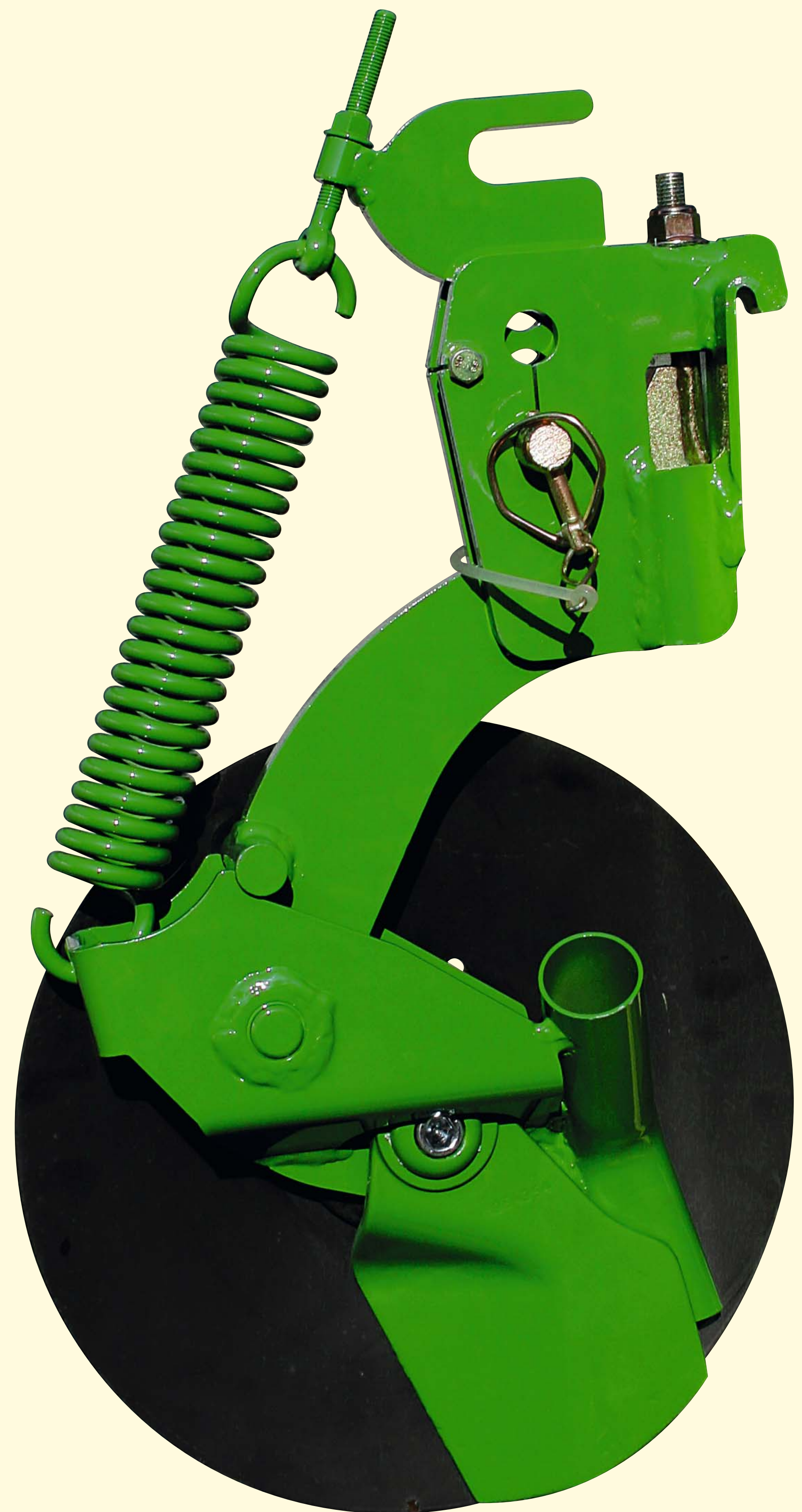
Scheibendüngerschare
