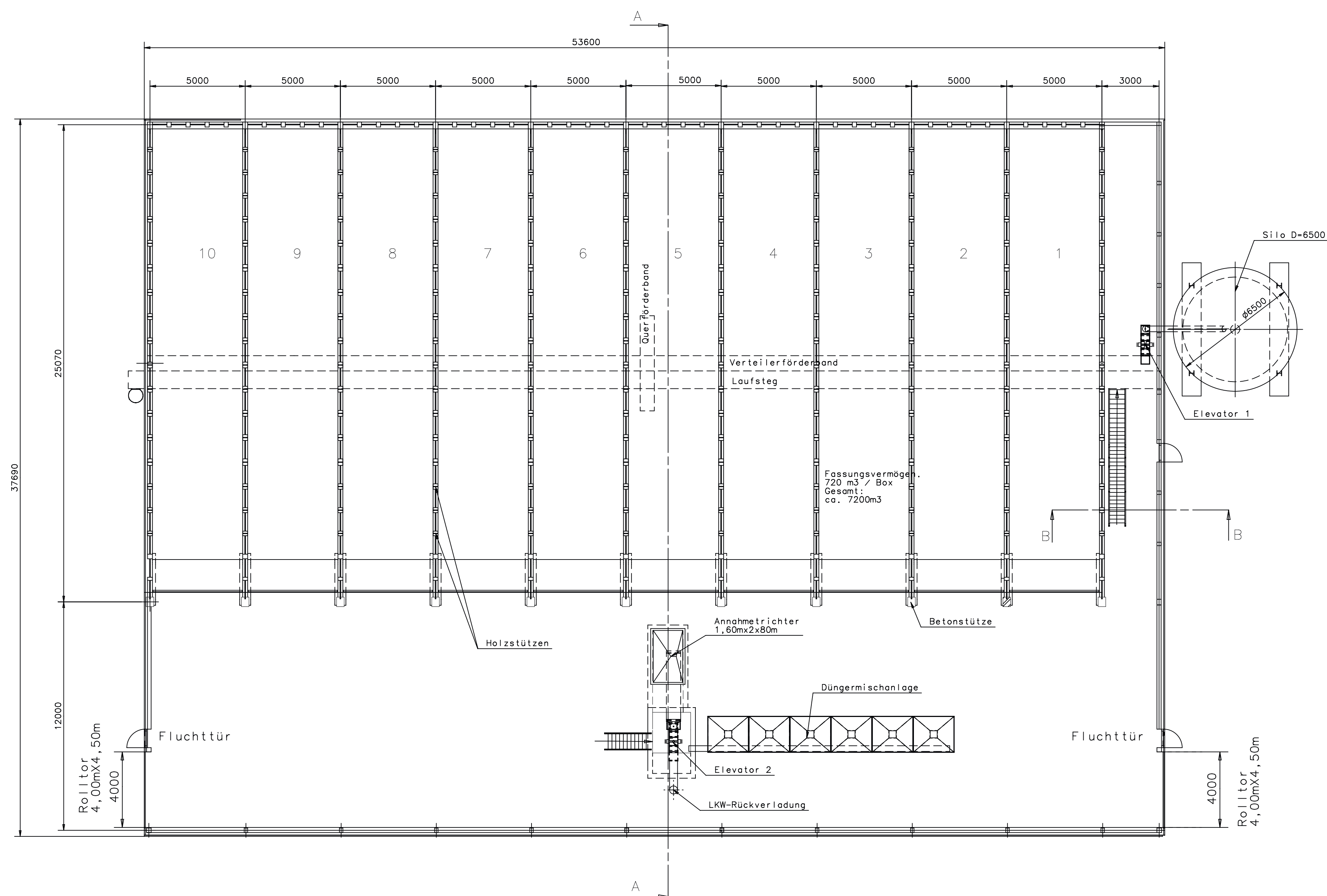
GRUNDRISS
