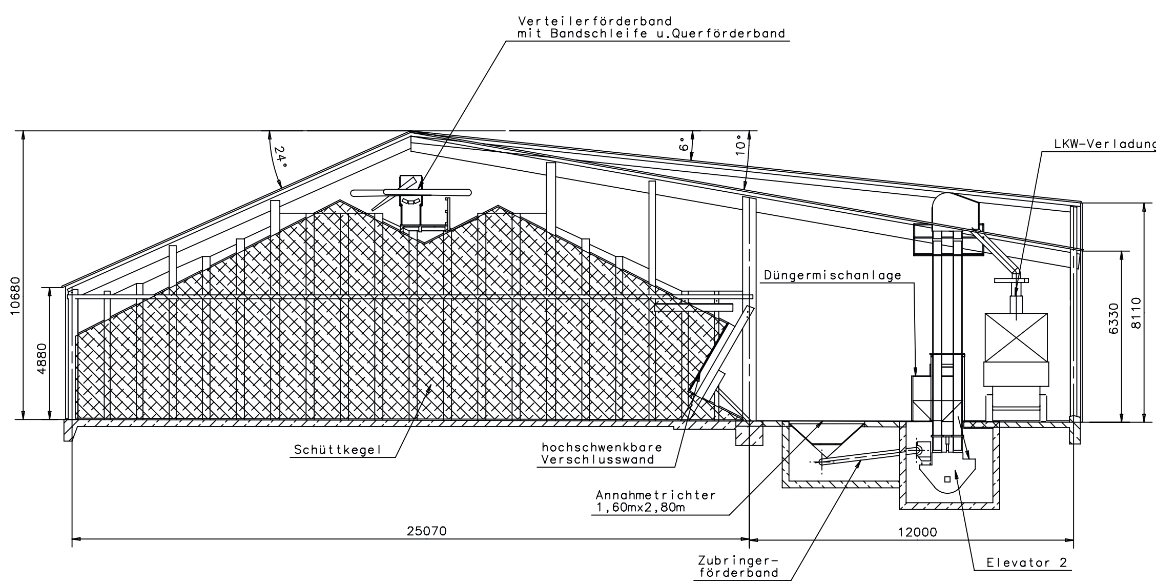
SCHNITT A-A
