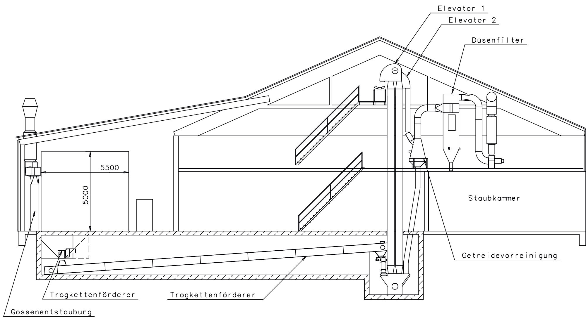
SCHNITT B-B
