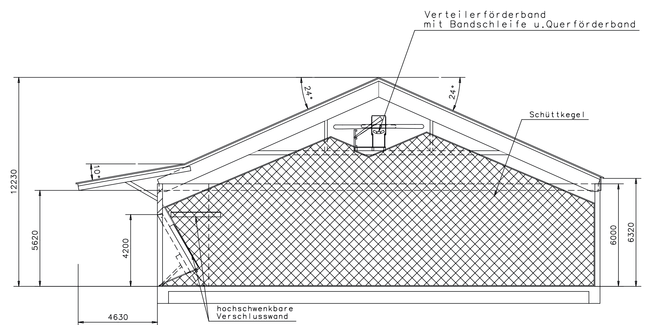
SCHNITT A-A
