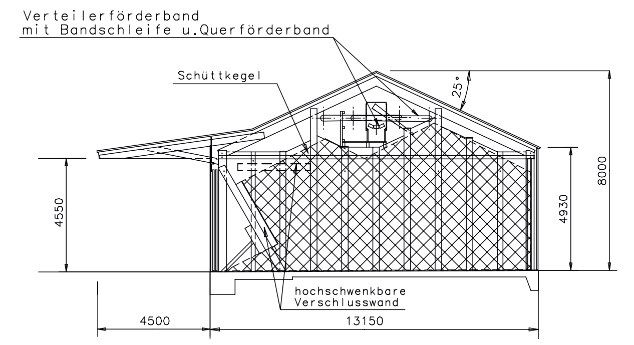
SCHNITT A-A
