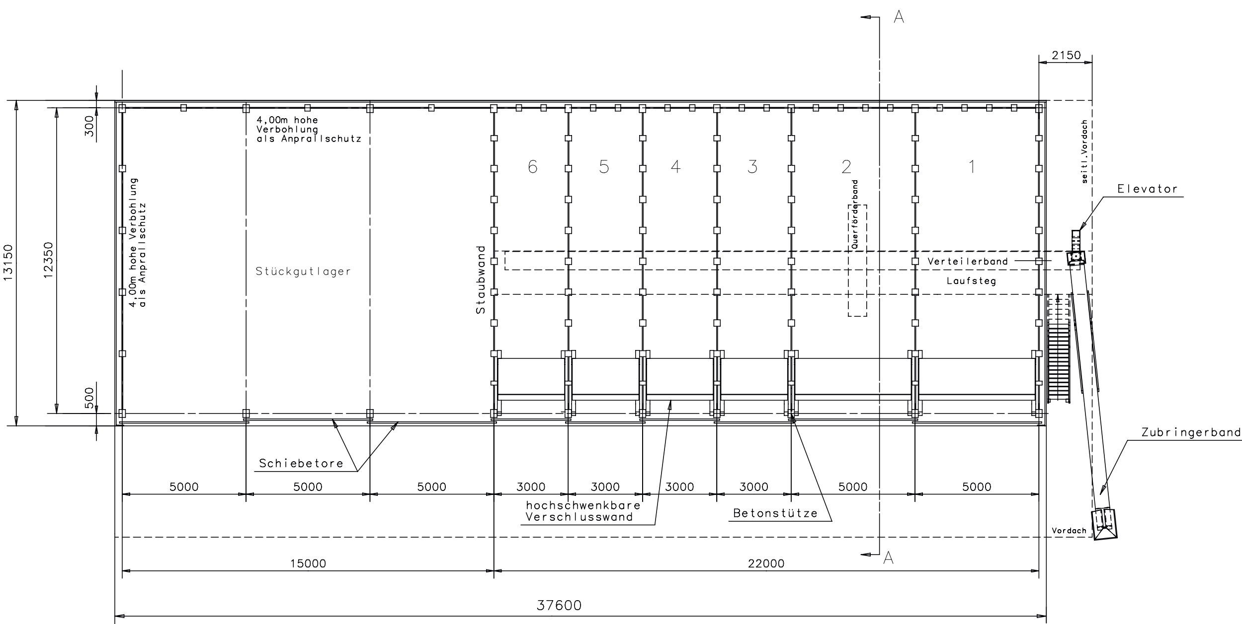
GRUNDRISS
