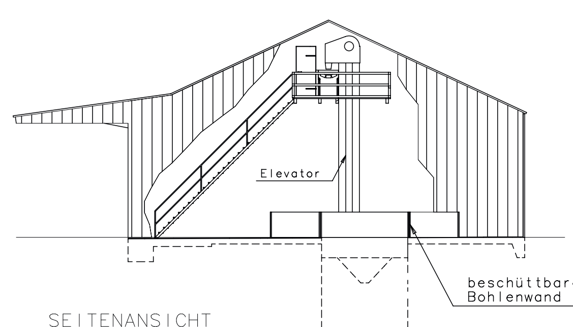
SEITENANSICHT
