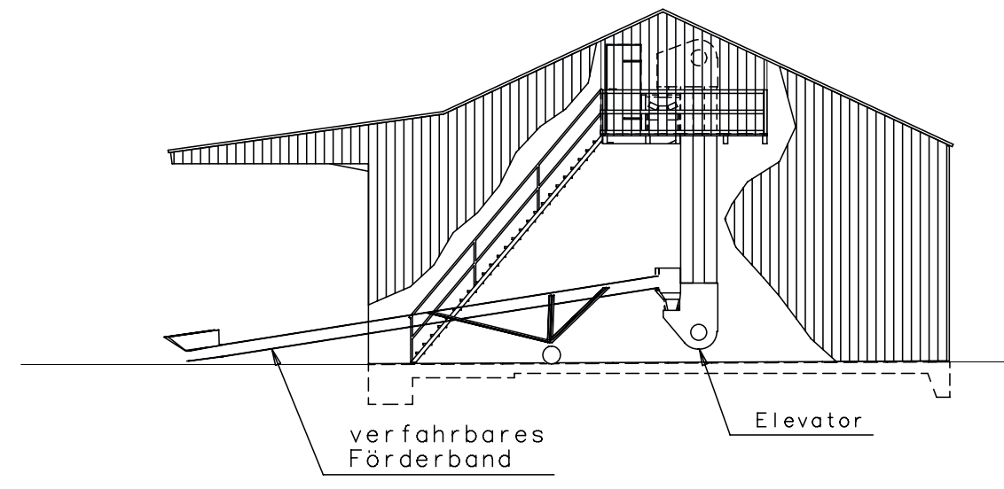
SEITENANSICHT
