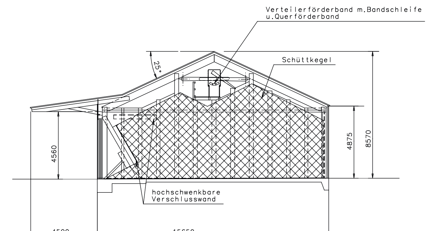
SCHNITT A-A
