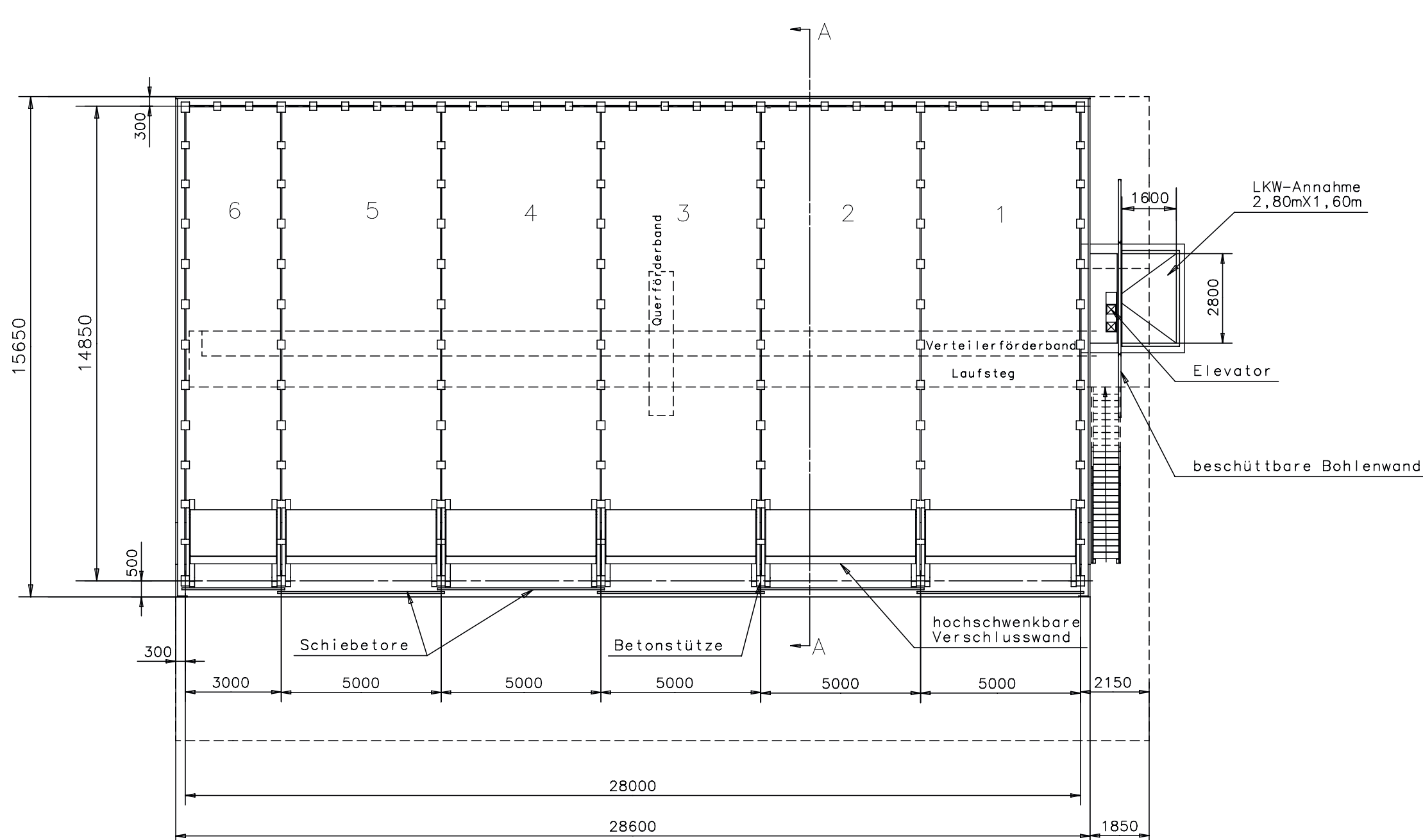
GRUNDRISS
