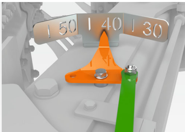
Hydraulisch instelling van de werkbreedte
