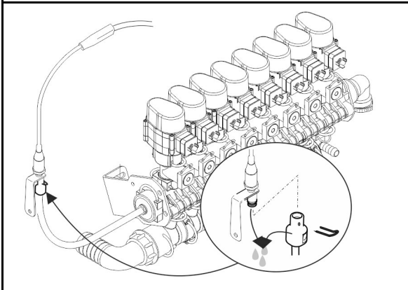
Spiediena sensors Super-L stieņi pie stieņu armatūras
