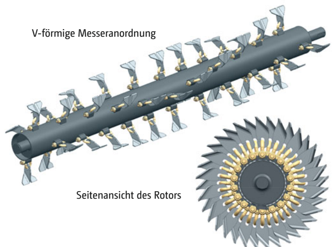
Exaktschnittrotor SmartCut
